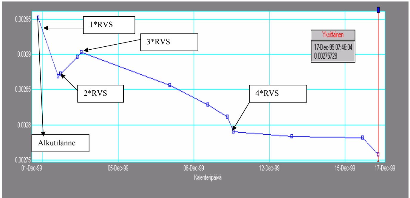
Kuvassa 6 nähdään moottorin ottaman virran muutos kokeen aikana
